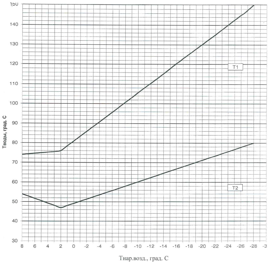
Рисунок 7 - Температурный график отпуса теплоты от Апатитской ТЭЦ на ЦТП г. Кировск
