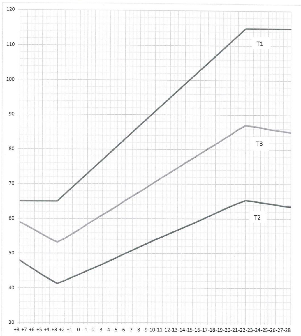
Рисунок 8 - Температурный график отпуски тепловой энергии от ЦТП г. Кировск
