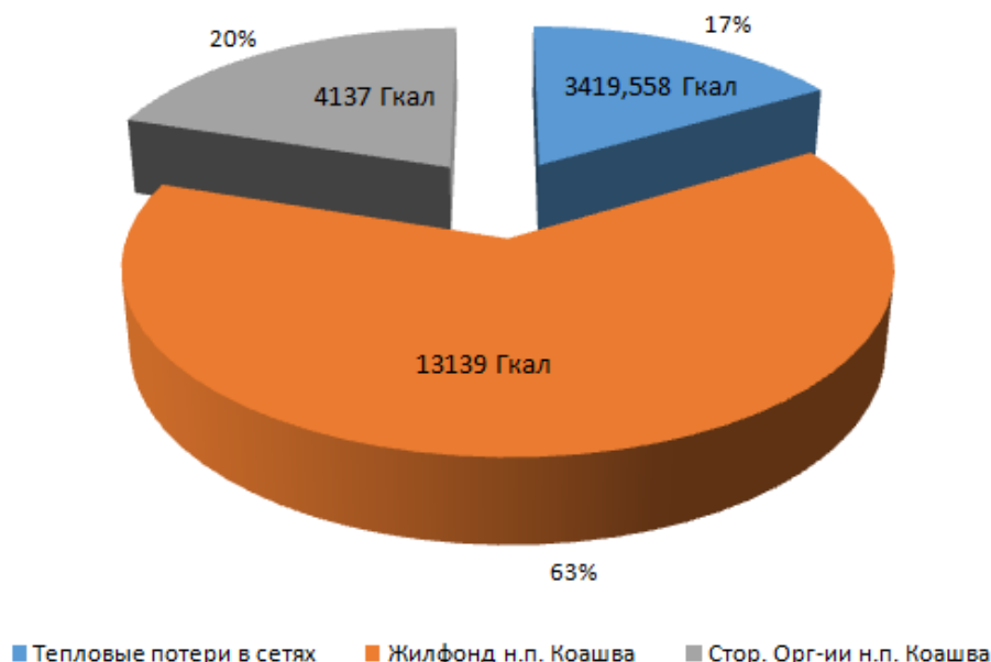
Рисунок 1.2.7 Структура выработки тепловой энергии автоматизированной блочно-модульной электростанцией н.п. Коашва
