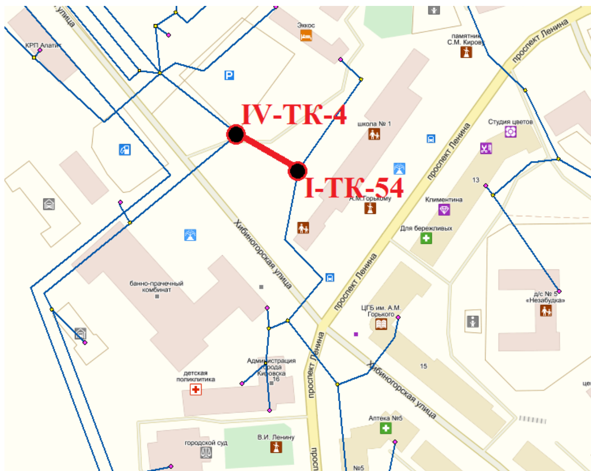
Рисунок 5.4.5 Схема предлагаемого к реконструкции участка тепловой сети В связи с изменением схемы трубопроводов мероприятия не актуально и его реализация не планируется.
