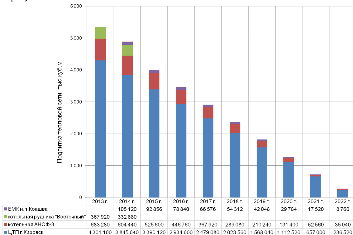
Рисунок 3.1.3 Ориентировочный план снижения годовых расходов подпиточной воды Средняя годовая экономия составит 564 тыс.м³/год. Что нарастающим итогом к 2022 году составит 5081 тыс.м³/год.
