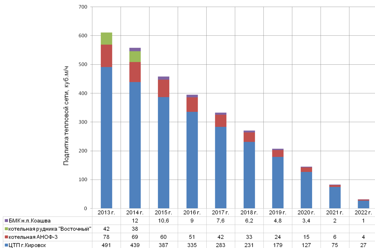
Рисунок 3.1.2 Ориентировочный план снижения часовых расходов подпиточной воды Ориентировочный план снижения годовых расходов подпиточной воды представлен на рисунке 3.1.3.
