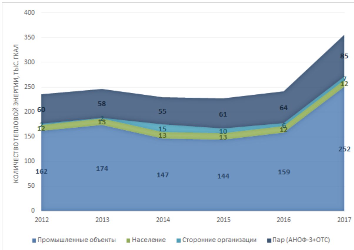
Рисунок 1.2.7 Потребление тепловой энергии с разделением по видам объекта
