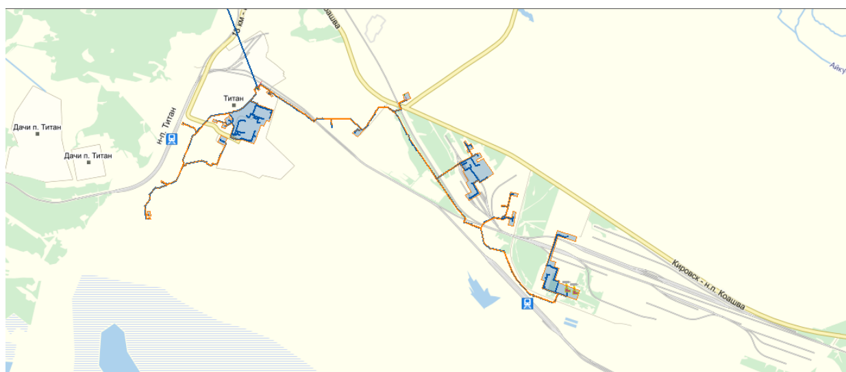
Рисунок 2.2.10 Зона действия системы теплоснабжения н.п. Титан и близлежащих промышленных площадок
