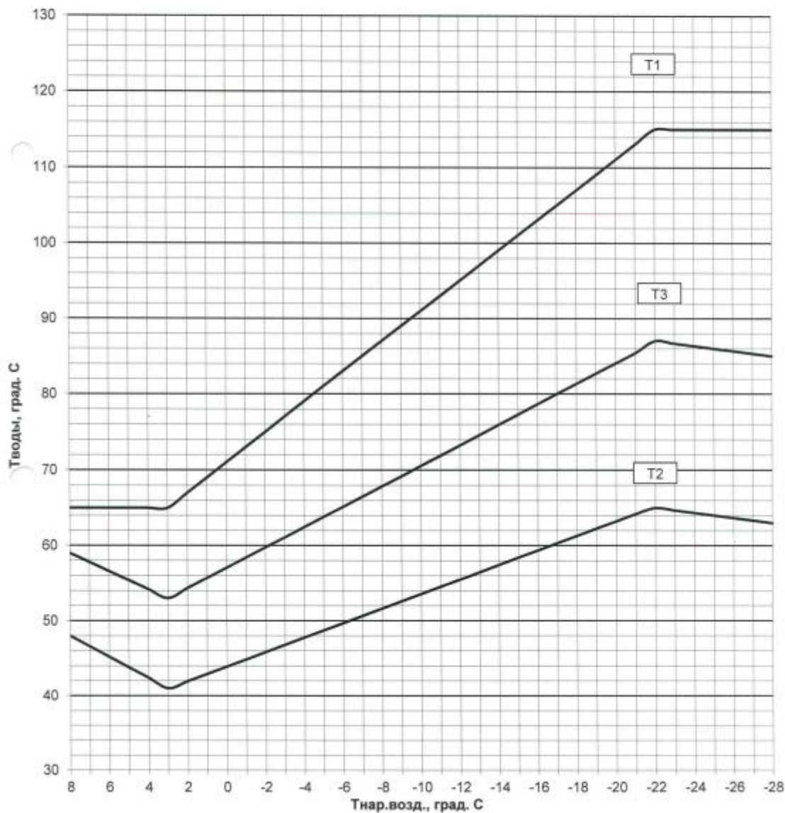
Рисунок 2.2.5 Температурный график работы ЦТП г. Кировска на отопительный сезон 2017-2018 гг.
