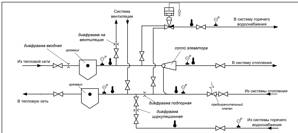
Рисунок 1.2.4 Принципиальная схема теплового узла потребителя
