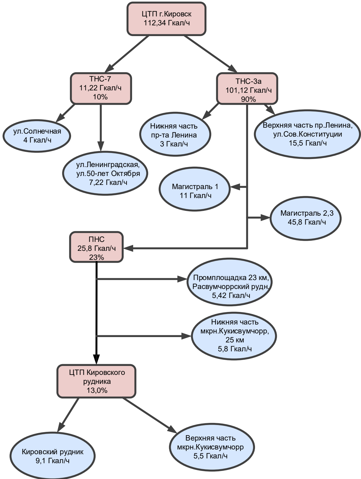
Рисунок 1.2.5 Схема распределения тепловой мощности от ЦТП
