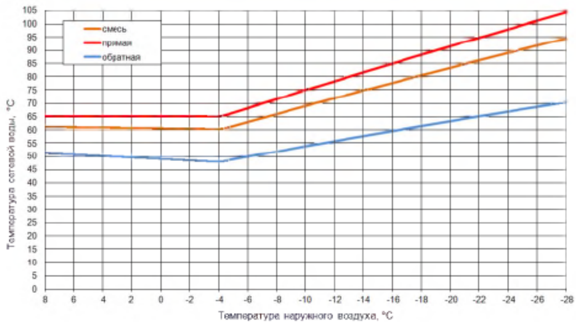
Температурный график электрической БМК н.п.Коашва
