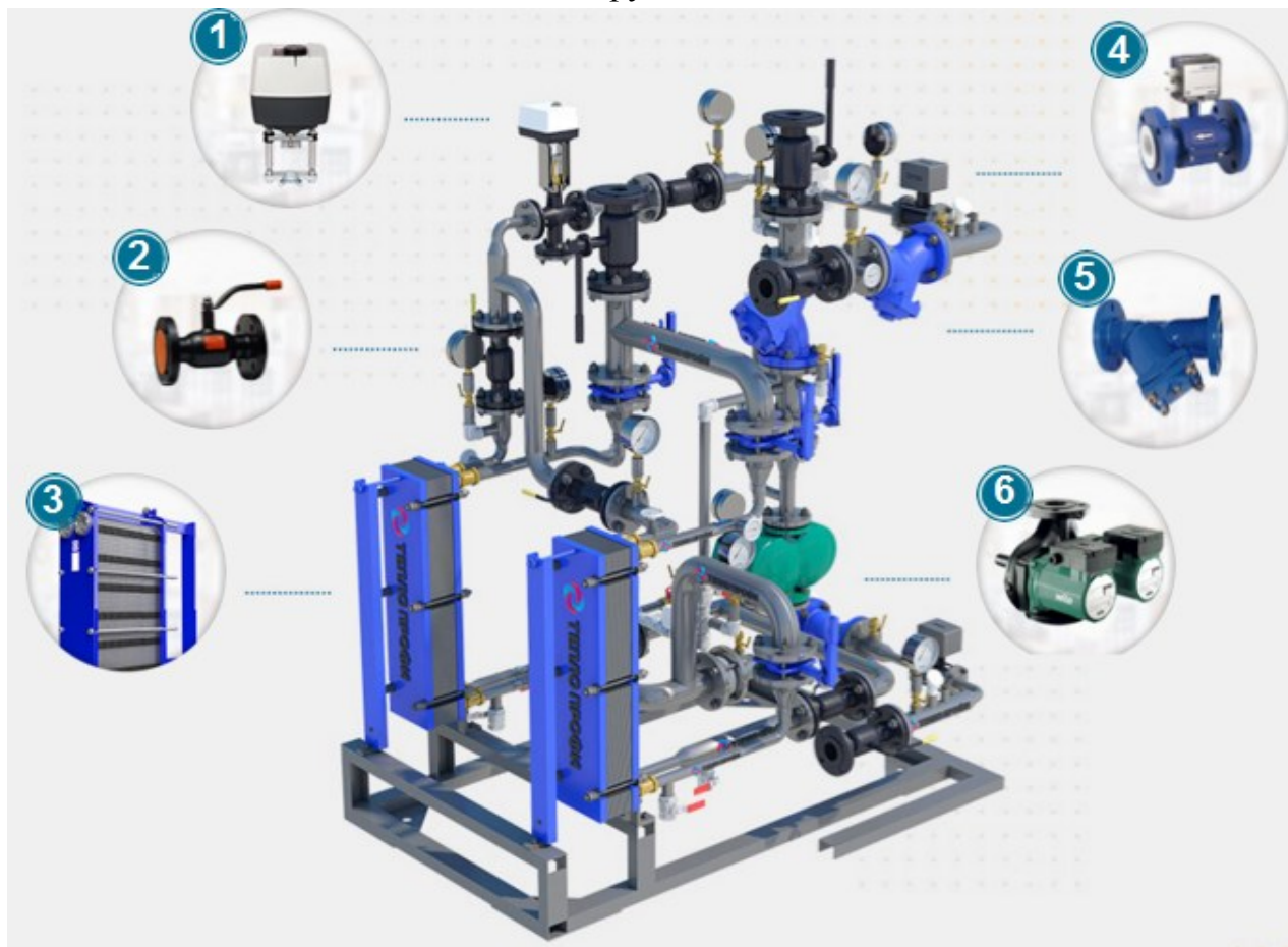
Оборудование ИТП
