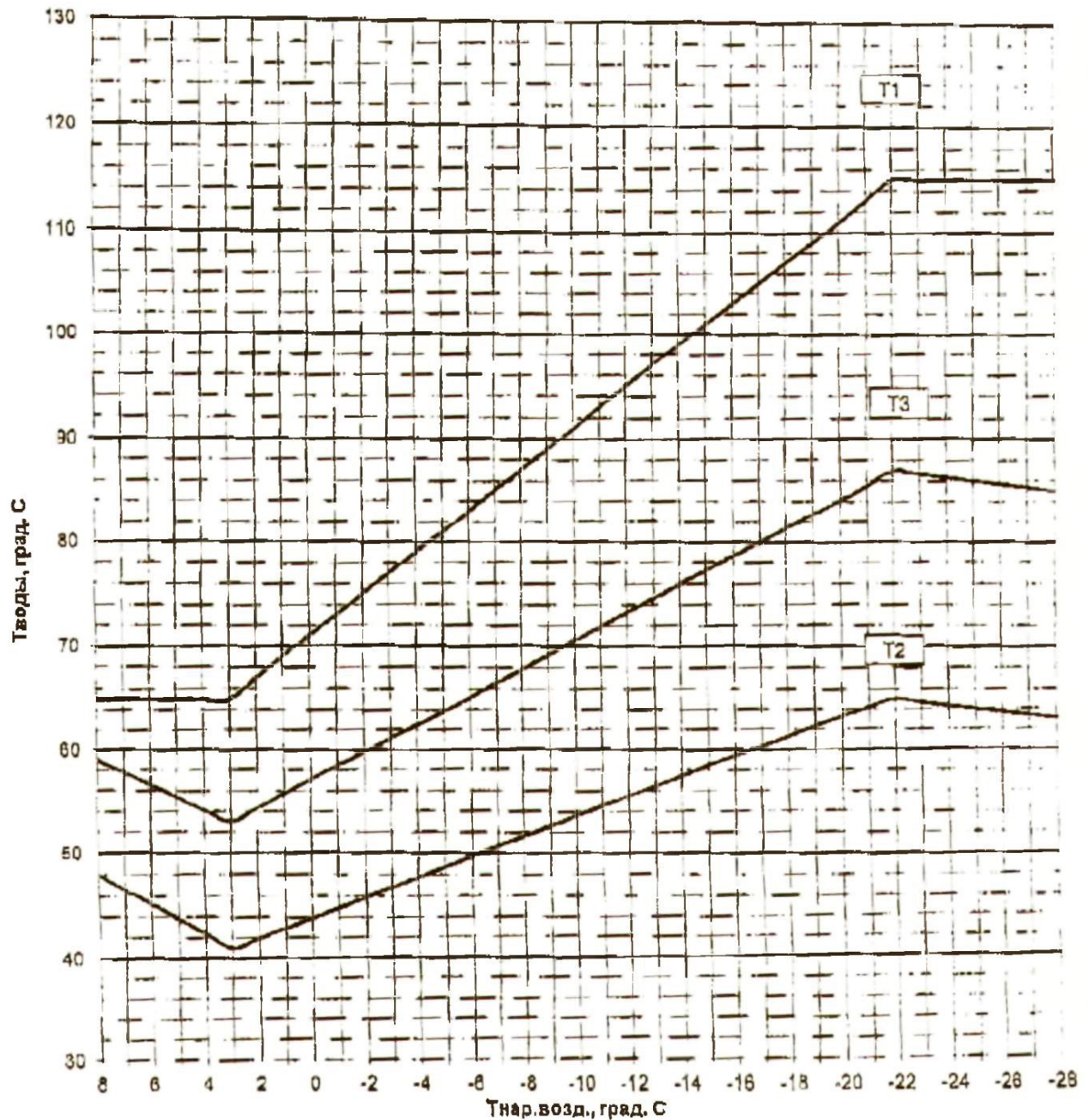
Рисунок 4.3 Температурный график работы тепловой сети от ЦТП г.Кировск
