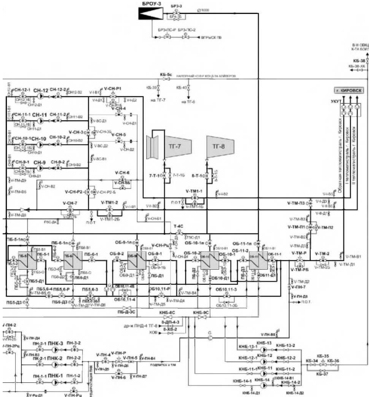
Рисунок 2.7 Схема блока теплофикационной установки на Апатитской ТЭЦ для г.Кировска
